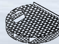
Impingement tray
